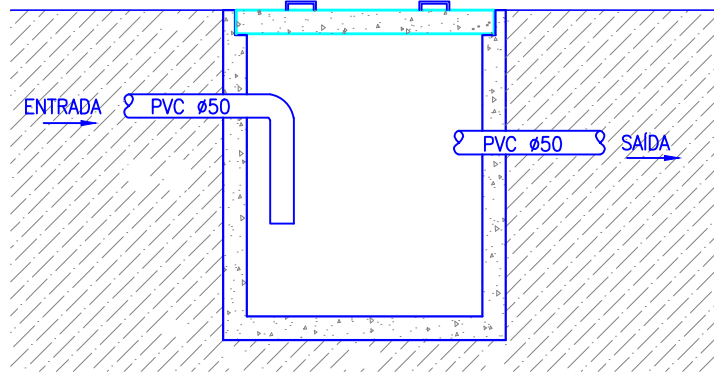
CORTE AA'
